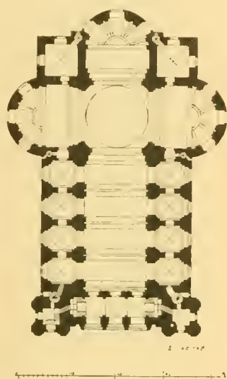
Fig. 1. Dom zu Salzburg. Grundriss
